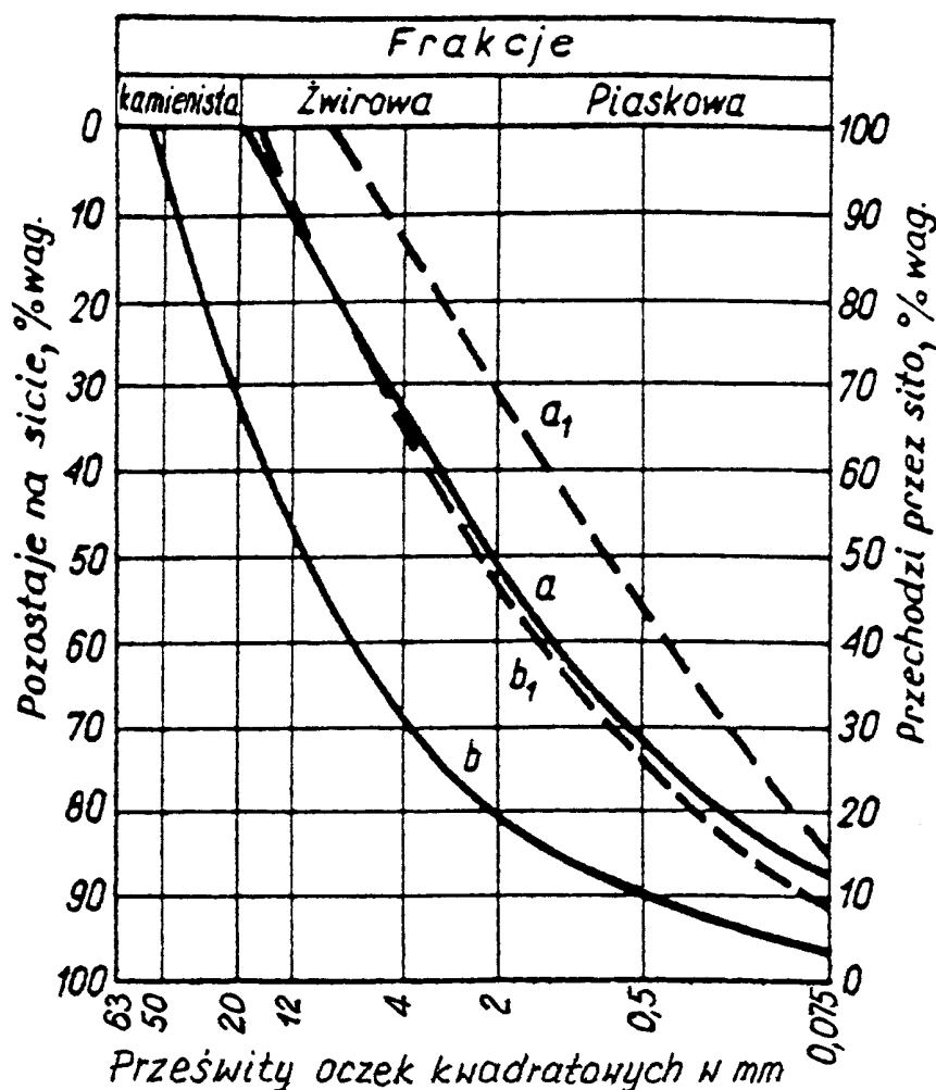
Obszar uziarnienia optymalnych mieszanek żwirowych
